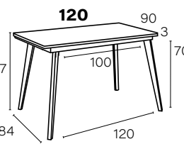
M811 Mesa EXTENSIBLE, patas metálicas INCLINADAS 300 PUNTOS
