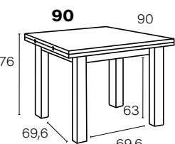
M901 Mesa EXTENSIBLE, patas CUADRADAS 172 PUNTOS
