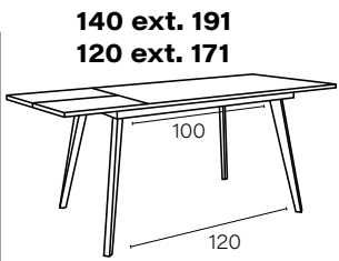
DETALLE MESA ABIERTA
