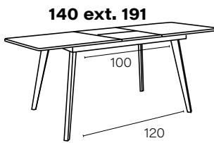
DETALLE MESA ABIERTA
