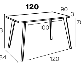
M813 Mesa FIJA, patas metálicas INCLINADAS 158 PUNTOS
