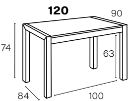
M607 Mesa EXTENSIBLE, patas PORTERÍA 333 PUNTOS
