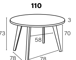
M817 Mesa FIJA, patas metálicas INCLINADAS 167 PUNTOS
