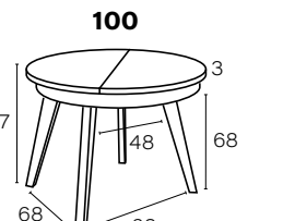
M816 Mesa EXTENSIBLE, patas metálicas INCLINADAS 308 PUNTOS
