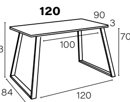
M803 Mesa FIJA, patas metálicas TRAPECIO 158 PUNTOS
