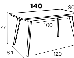
M810 Mesa EXTENSIBLE, patas metálicas INCLINADAS 308 PUNTOS
