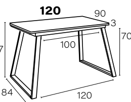
M801 Mesa EXTENSIBLE, patas metálicas TRAPECIO 300 PUNTOS
